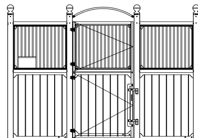
Vorderwand Luxe mit Tür in der Mitte
